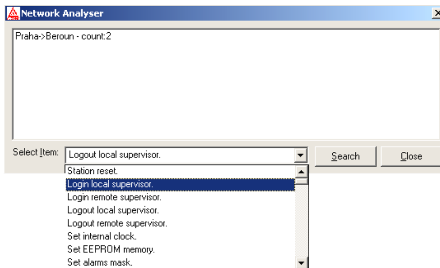
Obrázek 28 Prohlížení alarmů stanic
