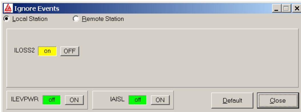
Obrázek 34 Nastavení masky událostí
