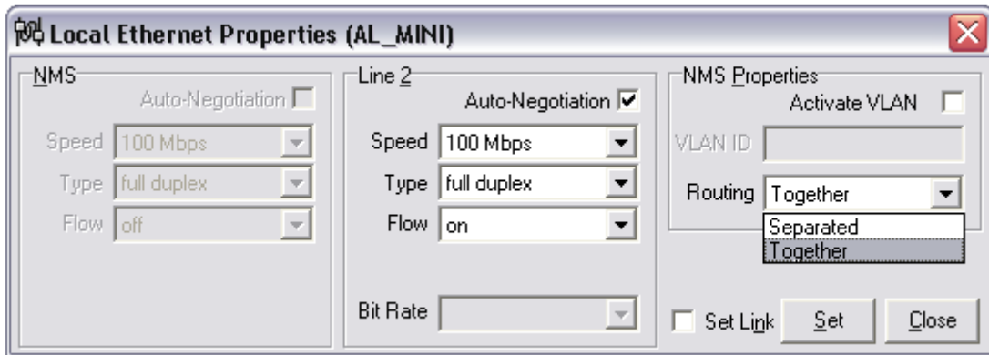
Obrázek 38 Nastavení přenosu Ethernetu
