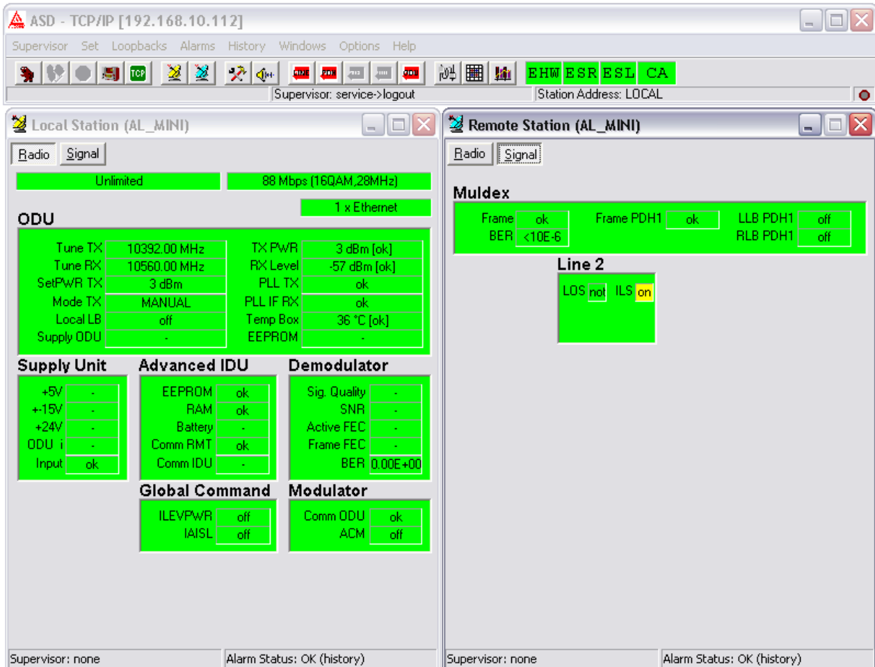
Obrázek 2 Okna zobrazení skoku spoje v lokálním módu dohledu
