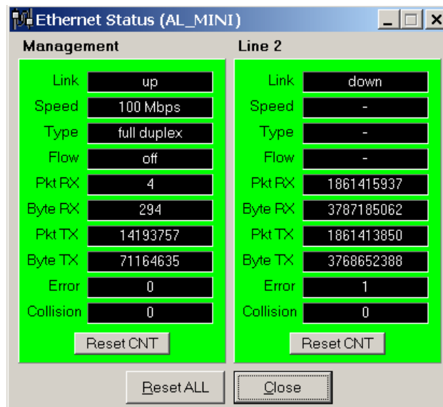
Obrázek 22 Okno stavu Ethernetu
