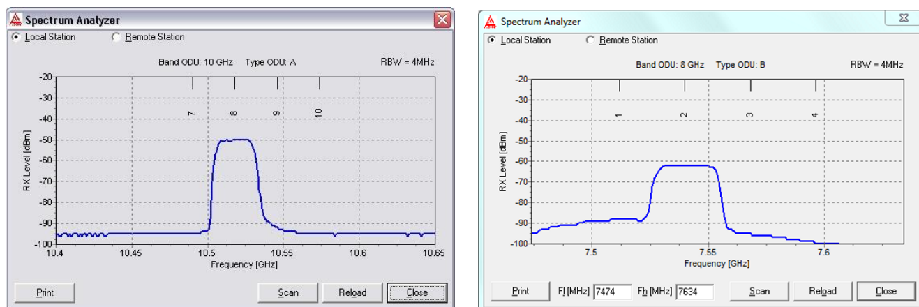
Obrázek 30 Spektrální analyzátor
