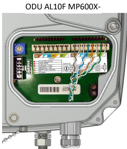
Obrázek 21 Dokončená montáž spojovacího kabelu Cat7 S-STP (1xGeth)
