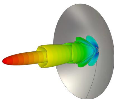
Obrázek 26 Vyzařovací charakteristika
