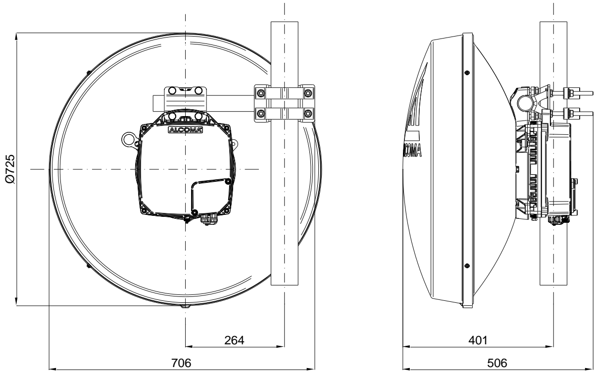
Obrázek 41 Hlavní rozměry stanice s anténou UNI2-10AS
