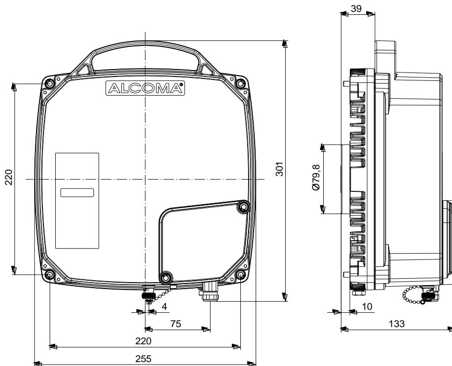
Obrázek 36 Hlavní rozměry ODU
