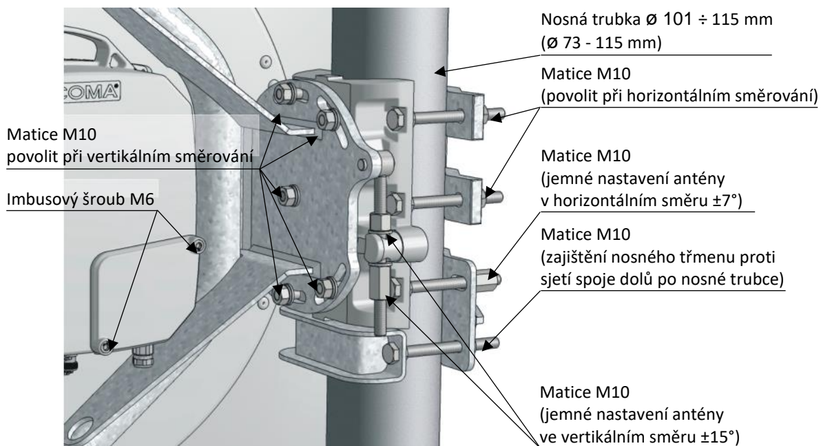
Obrázek 15 Uchycení držáku antény AL4-10/ME (také pro AL3-10/ME)
