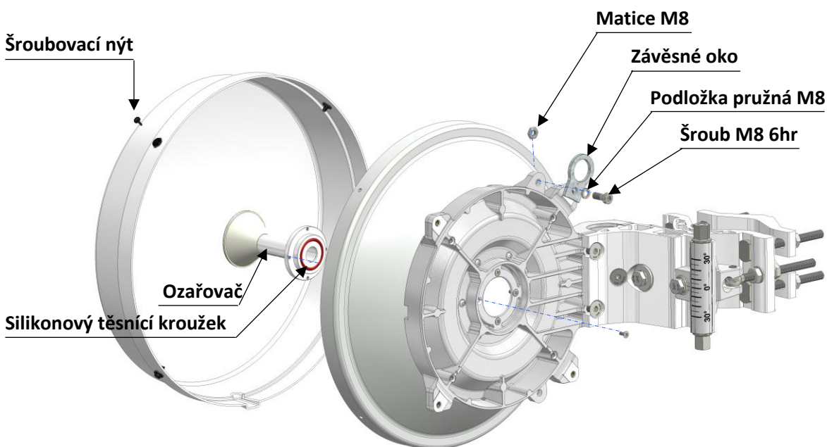
Obrázek 16 Připevnění ozařovače k anténě UNI1 (také pro UN2)
