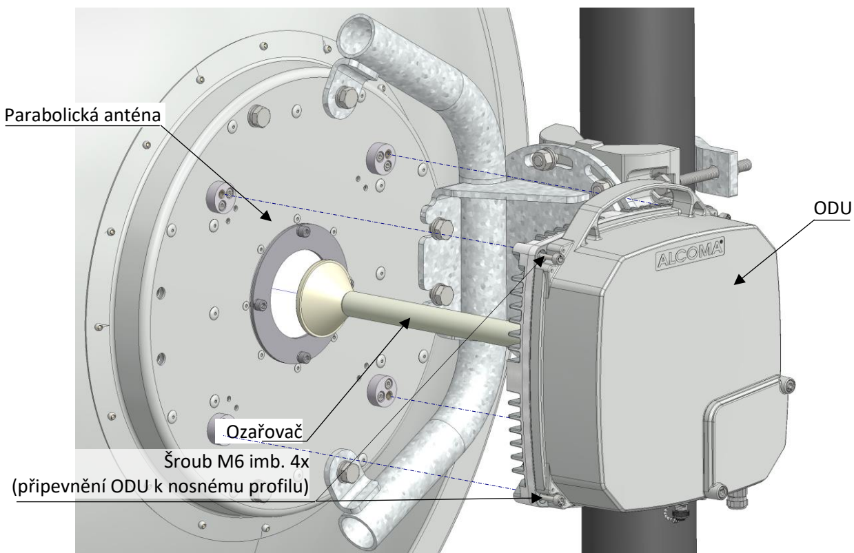
Obrázek 17 Montáž ODU na anténu AL3-10/ME (také pro AL4-10/ME)
