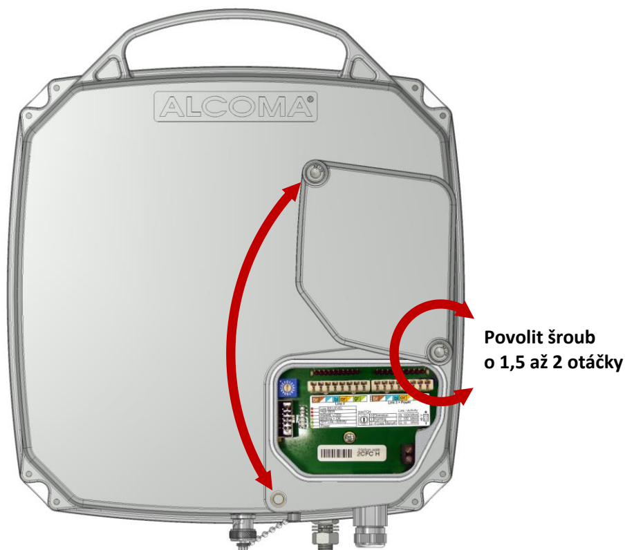
Obrázek 19 Manipulace s víčkem uživatelského prostoru
