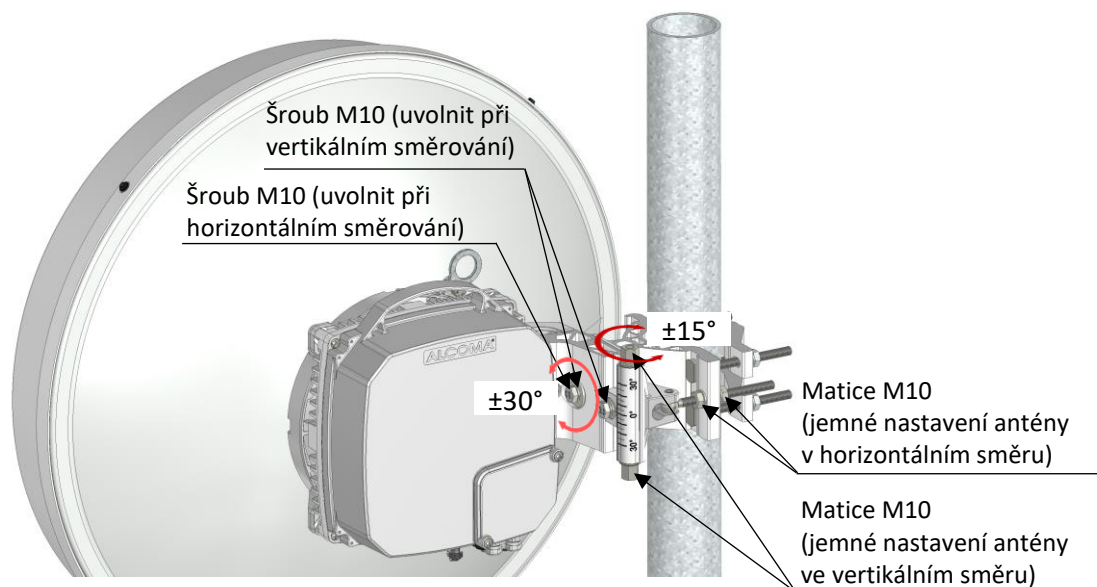
Obrázek 30 Směrování spoje s anténou typu UNI2-10AF (také pro UNI1-10AF)
