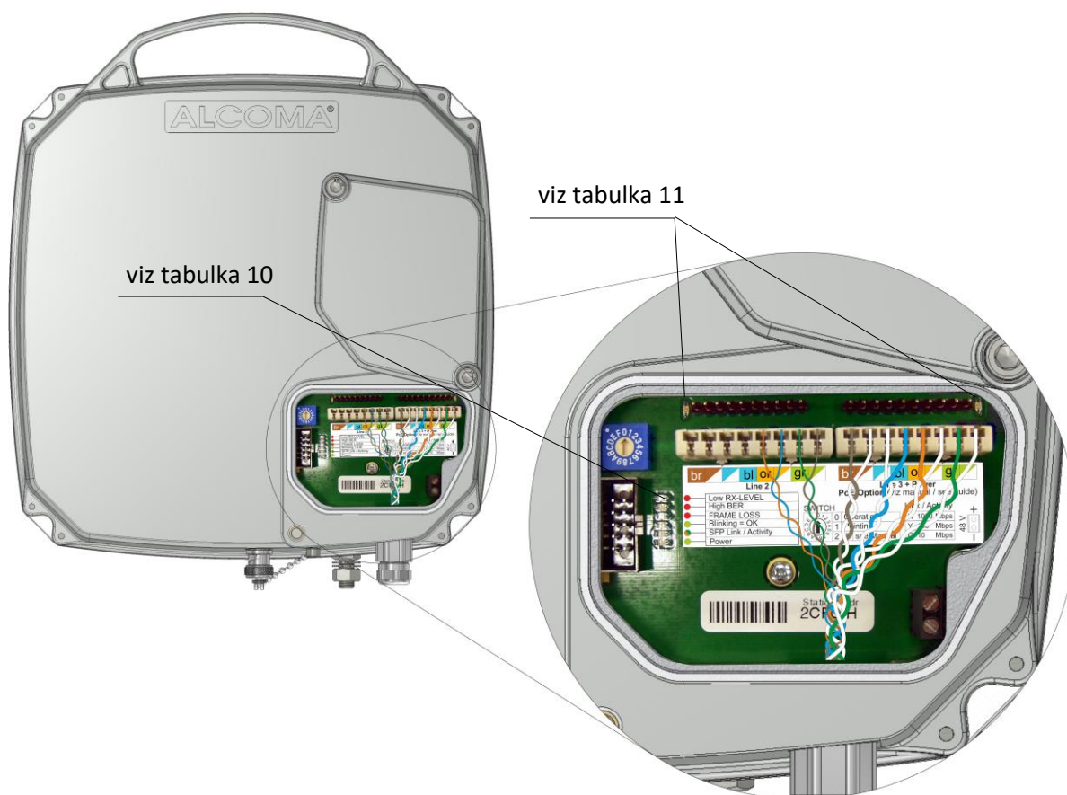
Obrázek 14 Uživatelský prostor ODU 1xGEth oddělený dohled
