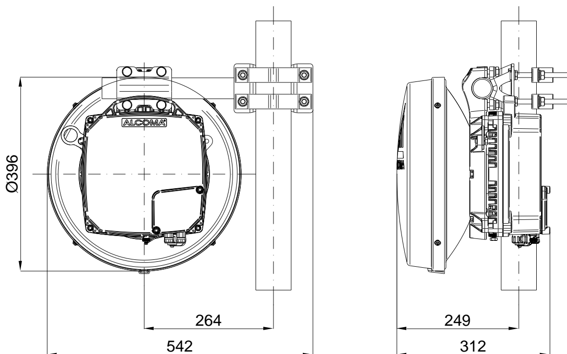
Obrázek 39 Hlavní rozměry stanice s anténou UNI1-10AS
