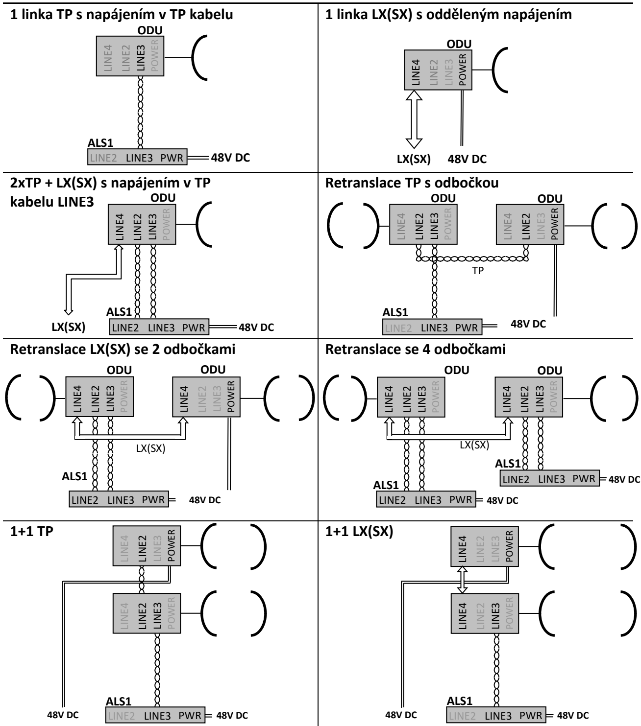
Obrázek 18 Typická zapojení ODU
