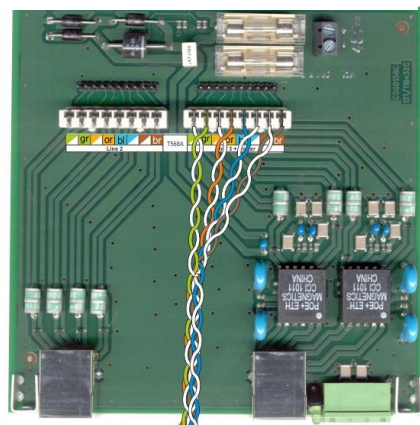
Chráněná svorkovnice ALS1-Geth
