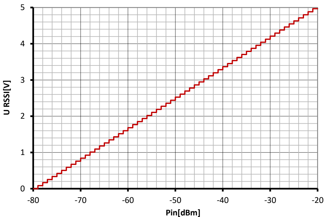
Obrázek 31 Kalibrační graf RSSI
