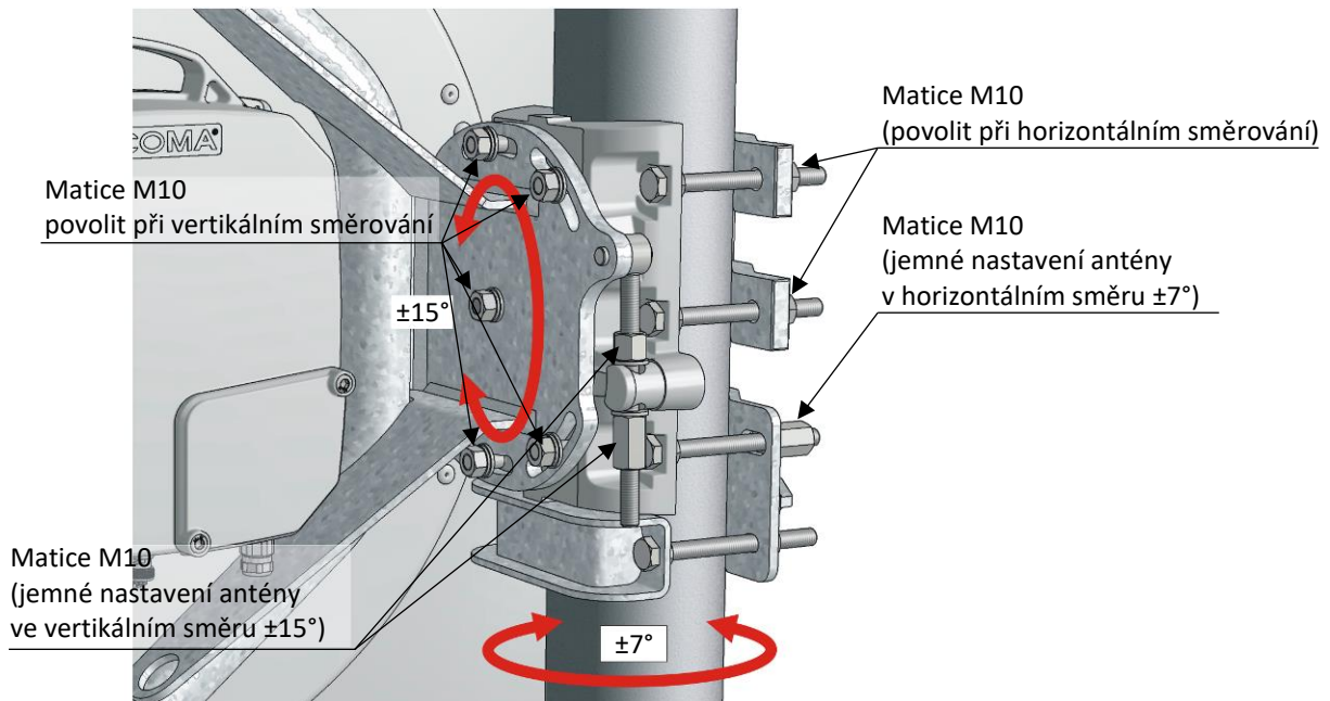
Obrázek 29 Směrování spoje s anténou typu AL4-10/ME (také pro AL3-10/ME)
