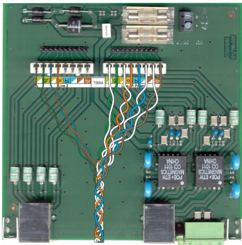
Obrázek 7 Oddělený dohled - zapojení kabelů ve svorkovnicích ALS1-GEth
