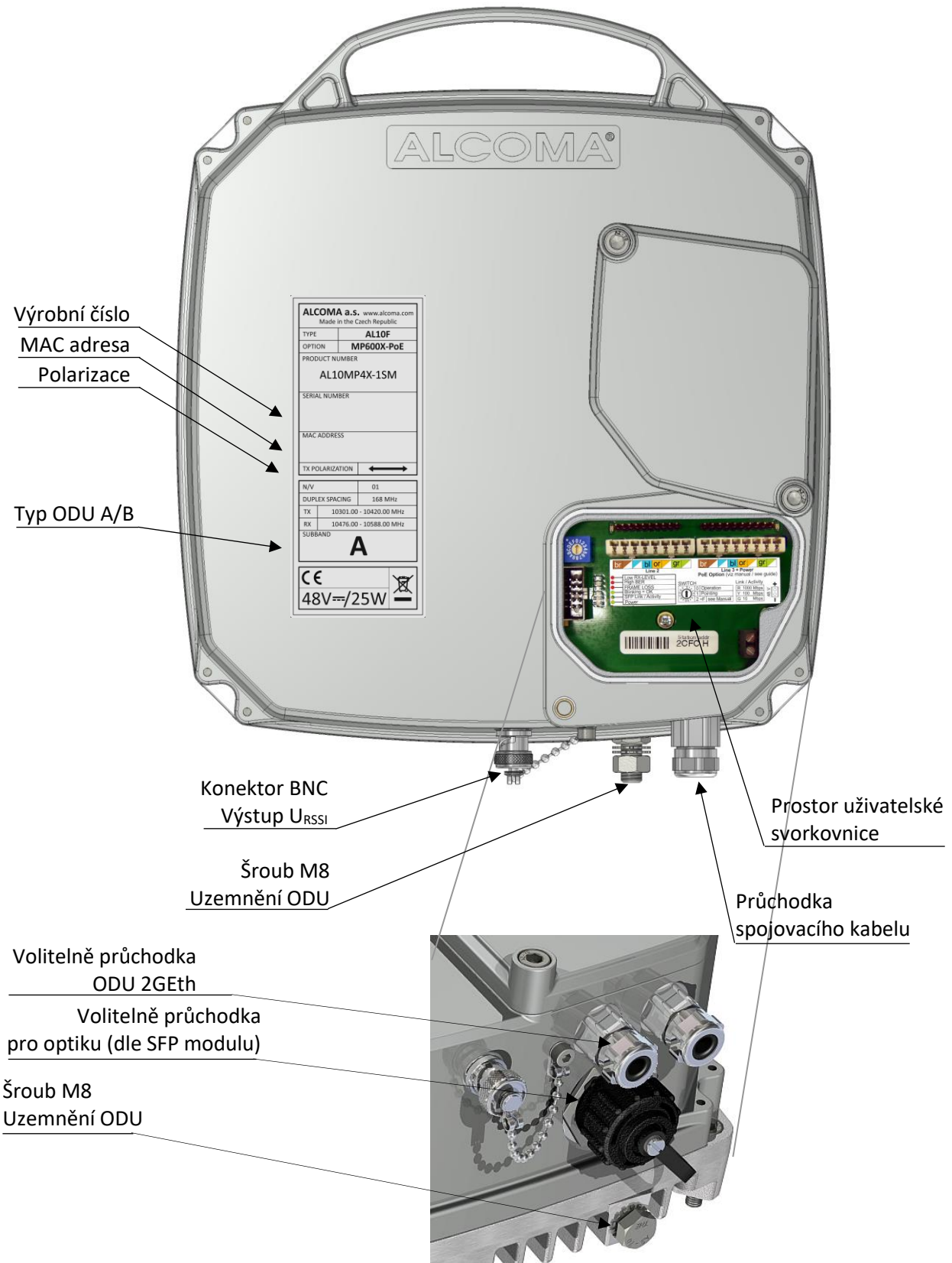
Obrázek 11 Připojná místa ODU
