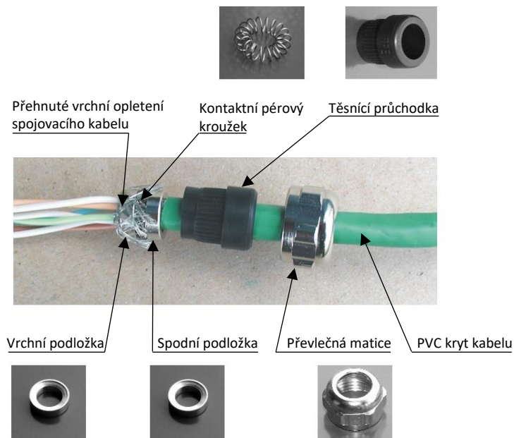
Obrázek 20 Montáž průchodky
