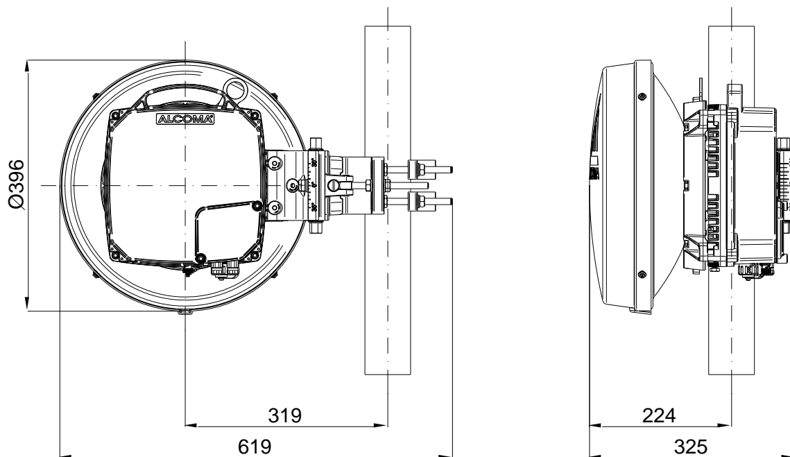
Obrázek 40 Hlavní rozměry stanice s anténou UNI1-10AF
