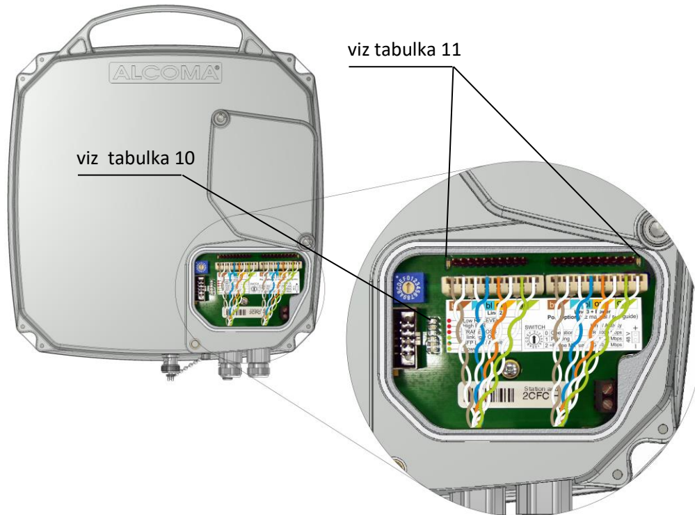
Obrázek 13 Uživatelský prostor ODU 2xGETh
