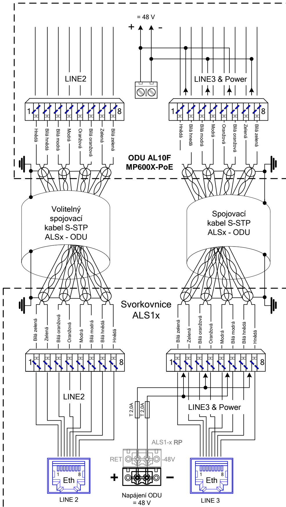
Obrázek 25 Připojení spojovacího kabelu
