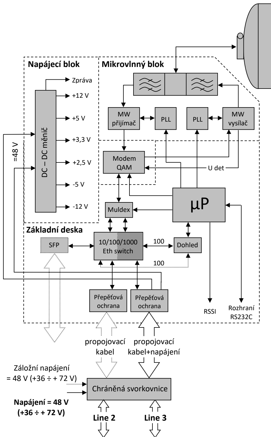
Obrázek 1 Blokové schéma spoje AL10F MP600X-PoE (Chráněná svorkovnice)
