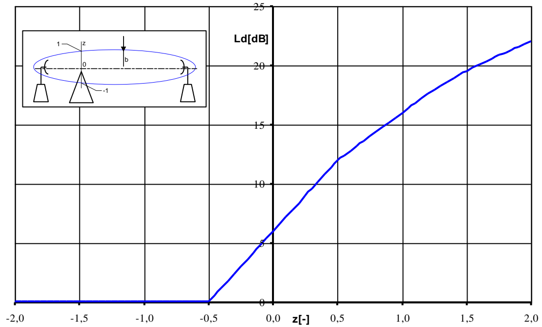
Obrázek 33 Aproximace přidavného útlumu za překážkou.
