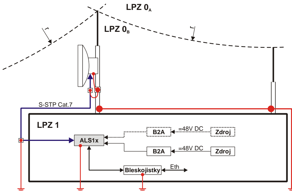
Obrázek 24 Uzemnění terminálu
