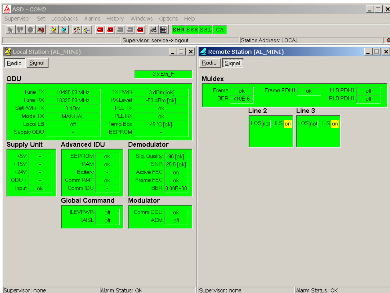
Obrázek 35 Hlavní okna programu ASD
