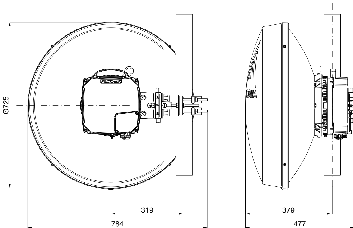
Obrázek 42 Hlavní rozměry stanice s anténou AL2-10AF
