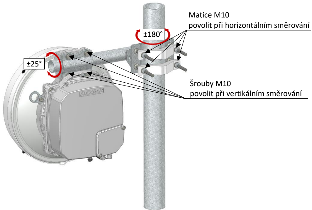
Obrázek 28 Směrování spoje s anténou typu UNI1-10AS (také pro UNI2-10AS)
