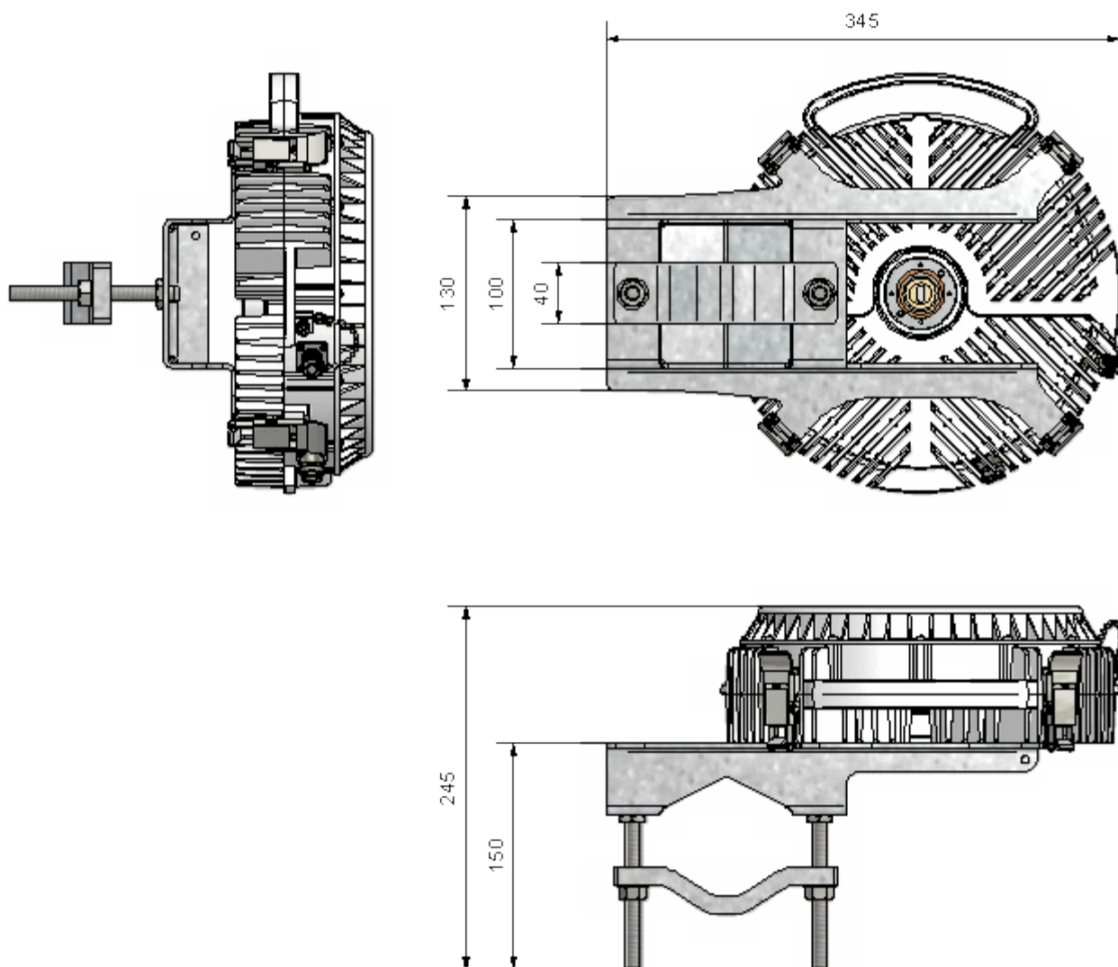
Obr. 7-2: Rozměry jednotky AL18F ODU s nosičem.
